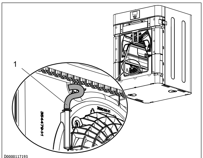
1 Tuyau antivibratoire
