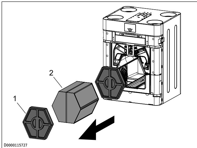
1 afstandshouder
