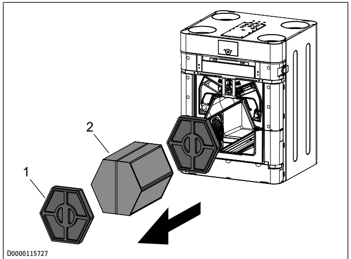
1 Entretroise 2 Échangeur de chaleur à flux croisé
